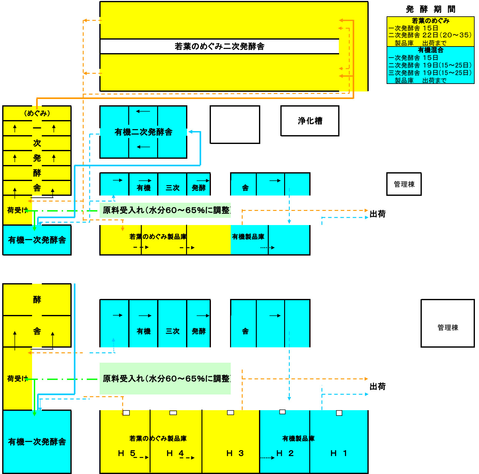
榊若葉 藤沢有機肥料センターフロー図(施設配置図)
